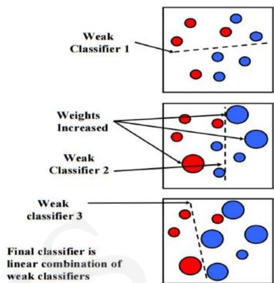
Fig. 3 AdaBoost[4]
